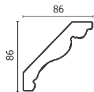
Молдинг 158-5
