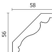
DD Карниз A1080-WG (58x56)
